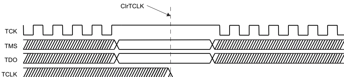
Figure 2-7. ClrTCLK
